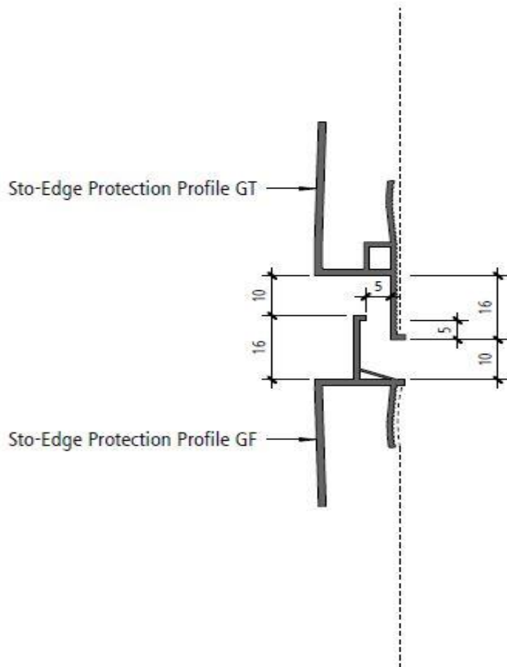
izvedba Sto-Kantenschutzprofil GT/GF
